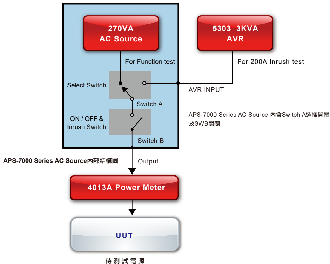
6010 ATE 使用 APS-7000 Series / 4013A 的結構圖
