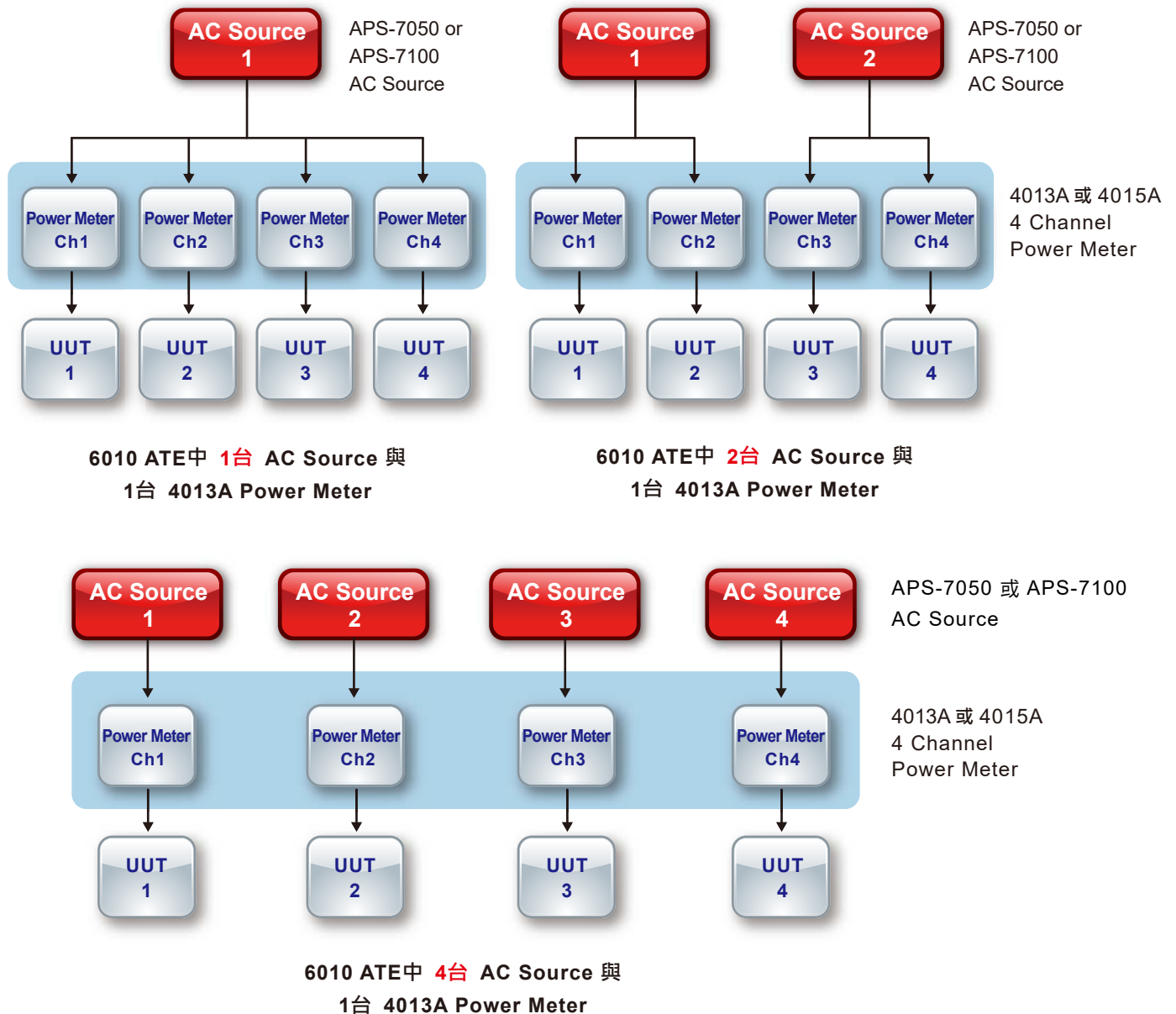
4013A 應用於6010 ATE配置圖
