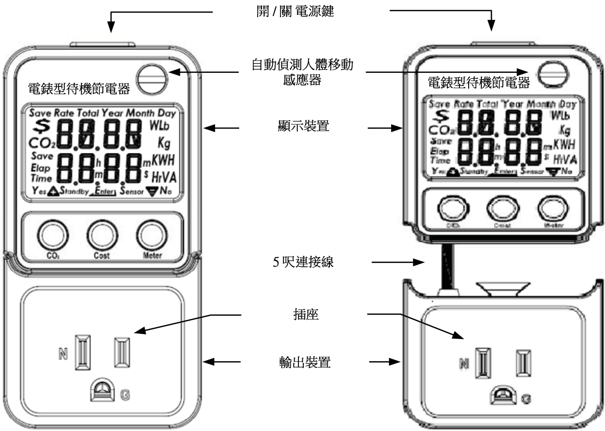
前面外觀圖
