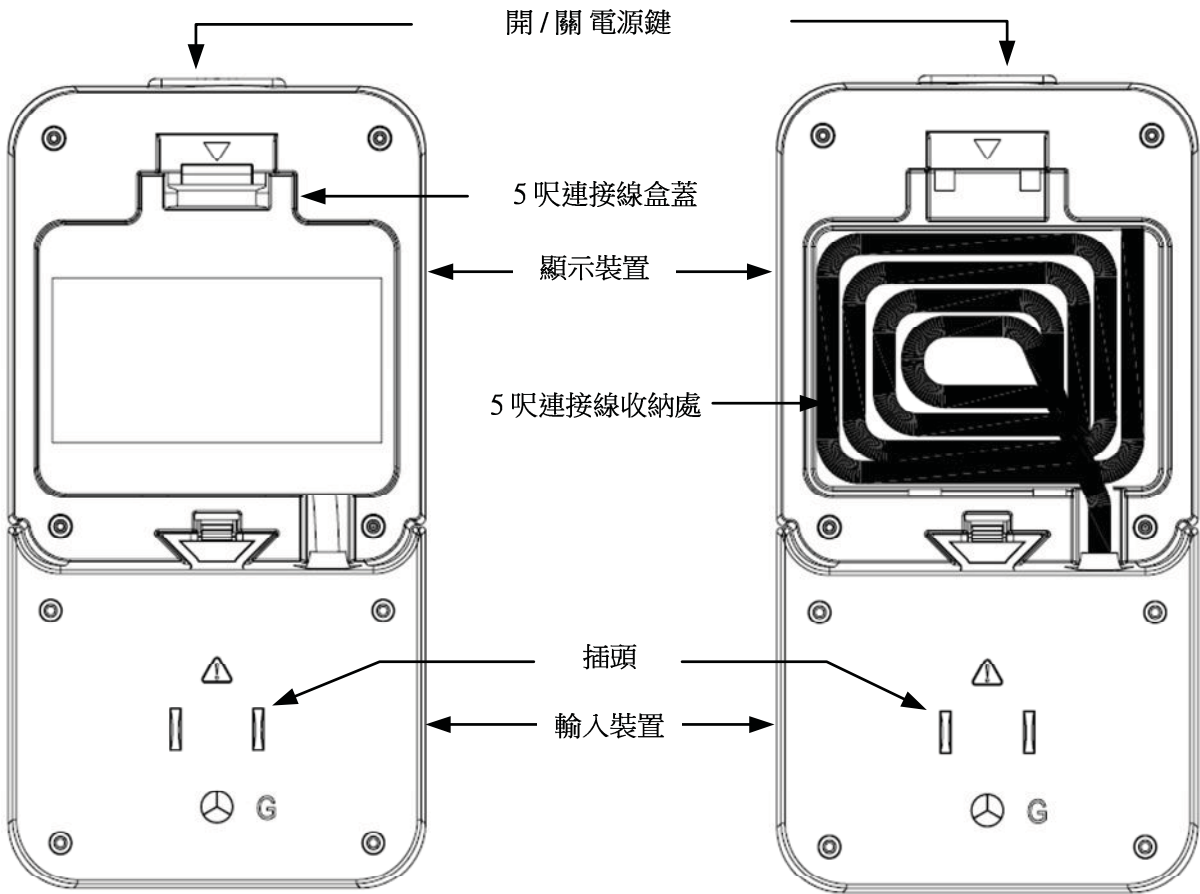
背面外觀圖
